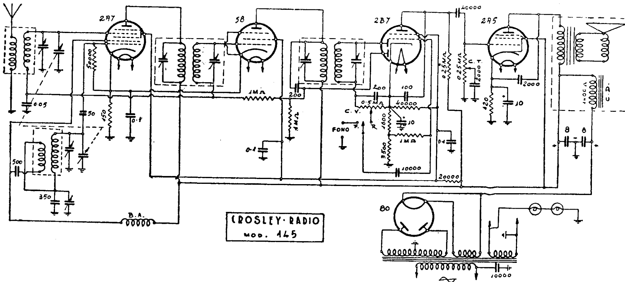
CROSLEY RADIO. — Modello « 145 ». - Produzione 1934. - Media frequenza: 350 kc.
